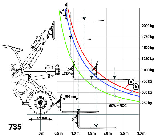
Belastningsdiagram 735
